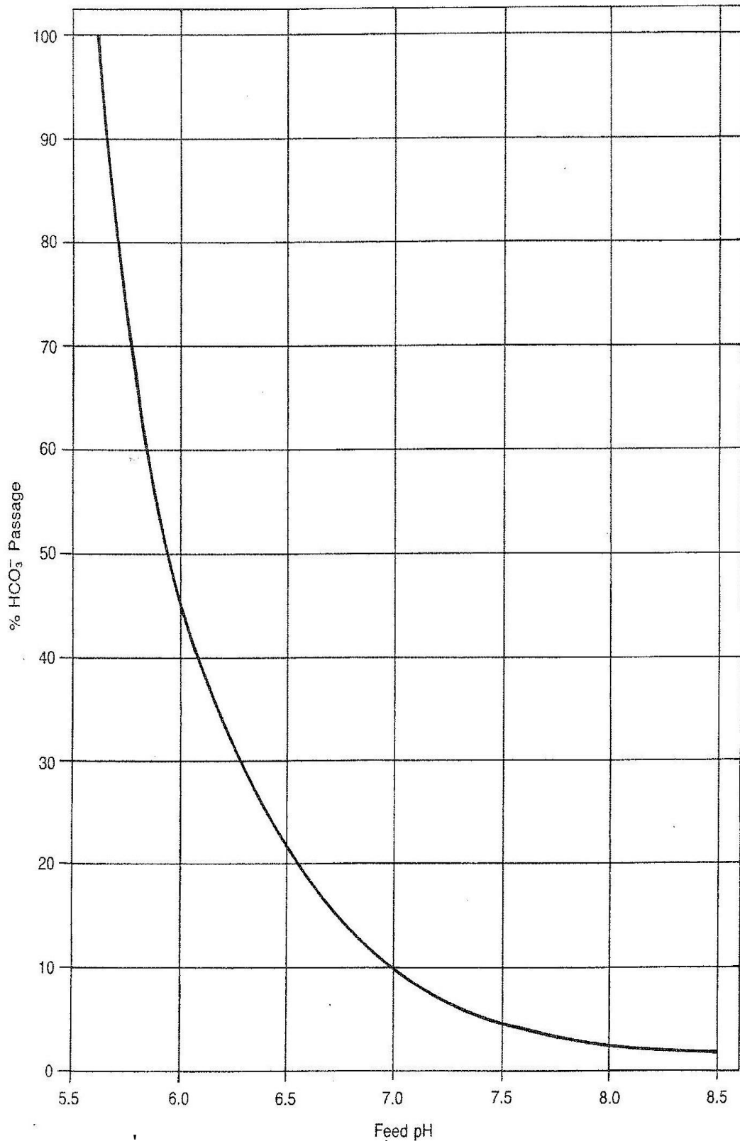
รูปที่ ๑ กราฟแสดงความสัมพันธ์ของ % \text{HCO}_3^- Passage และค่า Feed pH (Effect of Feed pH on \text{HCO}_3^- Passage for B-9 Permeator)
