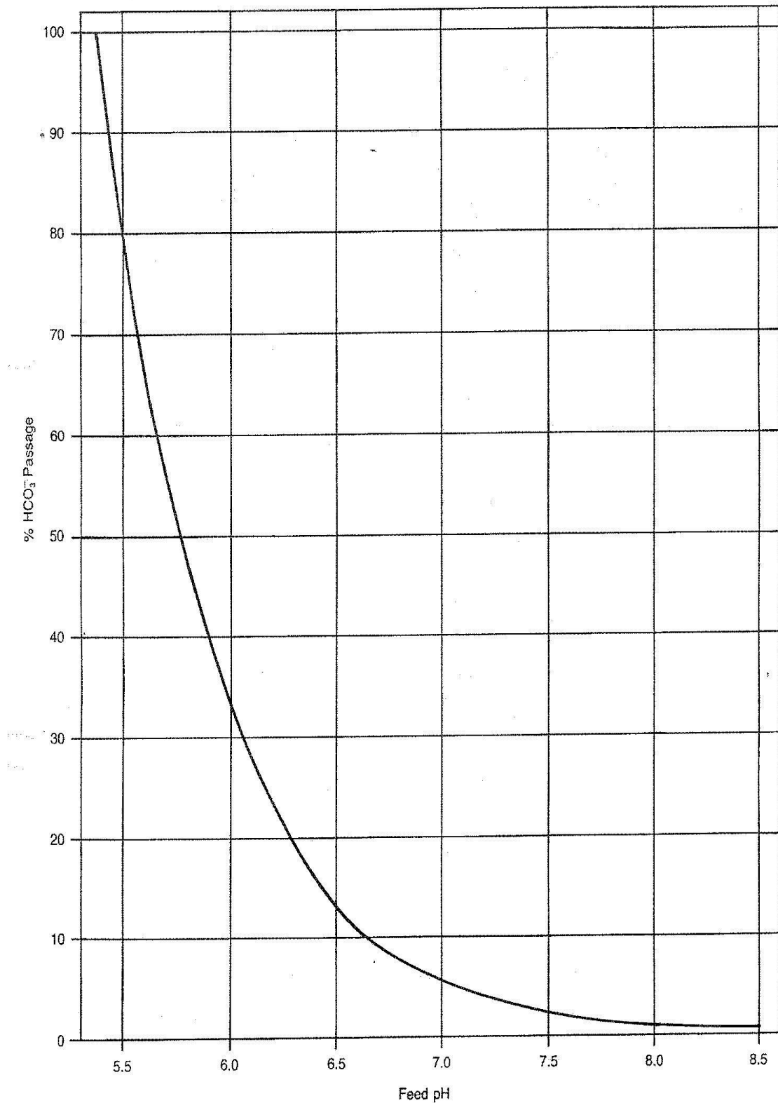
รูปที่ 10 กราฟแสดงความสัมพันธ์ของ % \text{HCO}_3^- Passage และค่า Feed pH (Effect of Feed pH on \text{HCO}_3^- Passage for B-10 Permeator)
