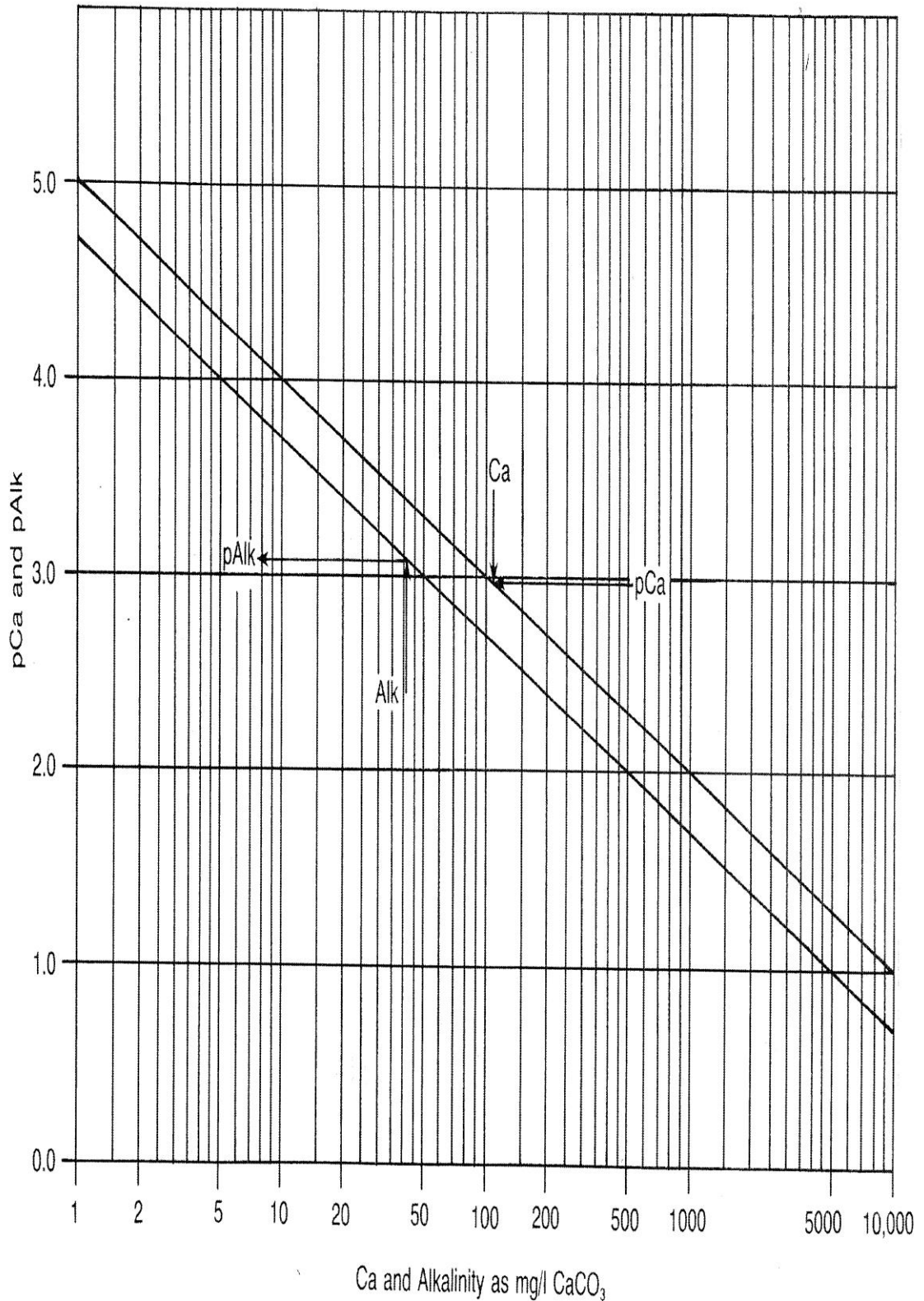
รูปที่ 8 กราฟความสัมพันธ์ของค่า pCa and pAlk และค่า Ca and Alkalinity as mg/l \text{CaCO}_3 (Conversion of Calcium and Alkalinity to pCa and pAlk)
