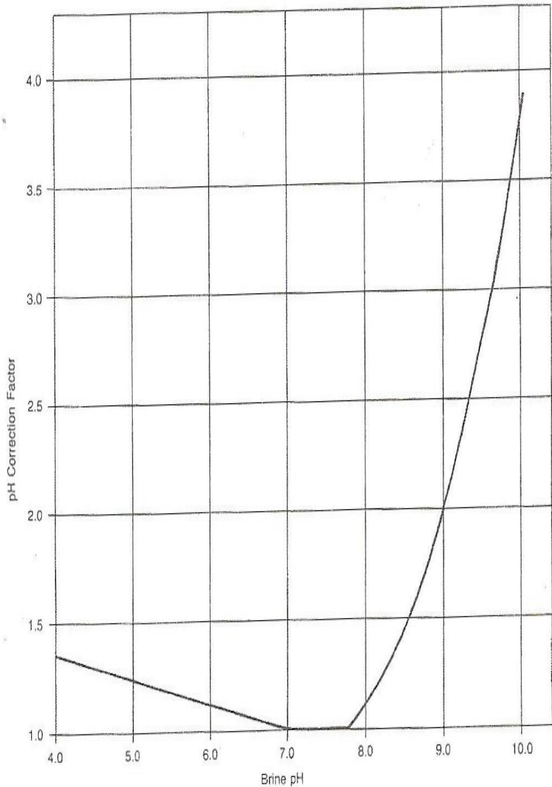
รูปที่ 14 กราฟแสดงความสัมพันธ์ของค่า pH Correction Factor และค่า Brine pH ( \text{SiO}_2 pH Correction Factor)
